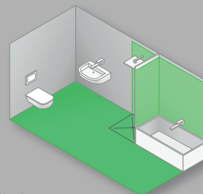
Häusliches Bad mit – Badewanne ohne Brause – bodengleicher Dusche ohne Duschabtrennung
