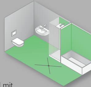
Häusliches Bad mit – Badewanne ohne Brause – Dusche mit Duschtasse und Duschabtrennung – Bodenablauf im Raum
